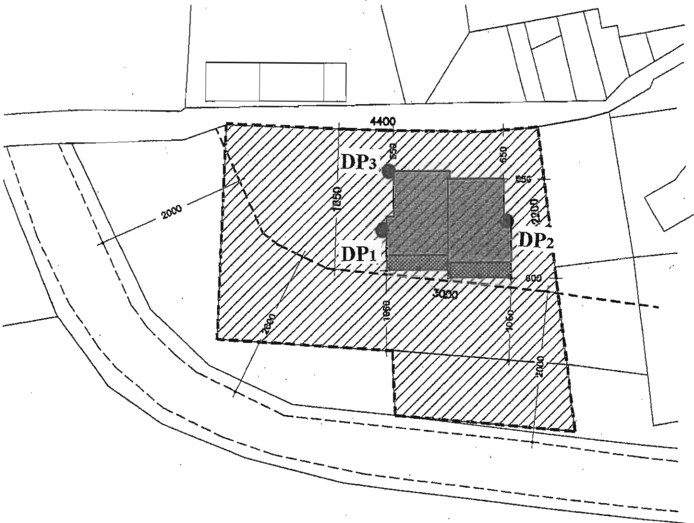
PLANIMETRIA DI PROGETTO IN SCALA 1 : 500 CON UBICAZIONE DELLE PROVE PENETROMETRICHE
