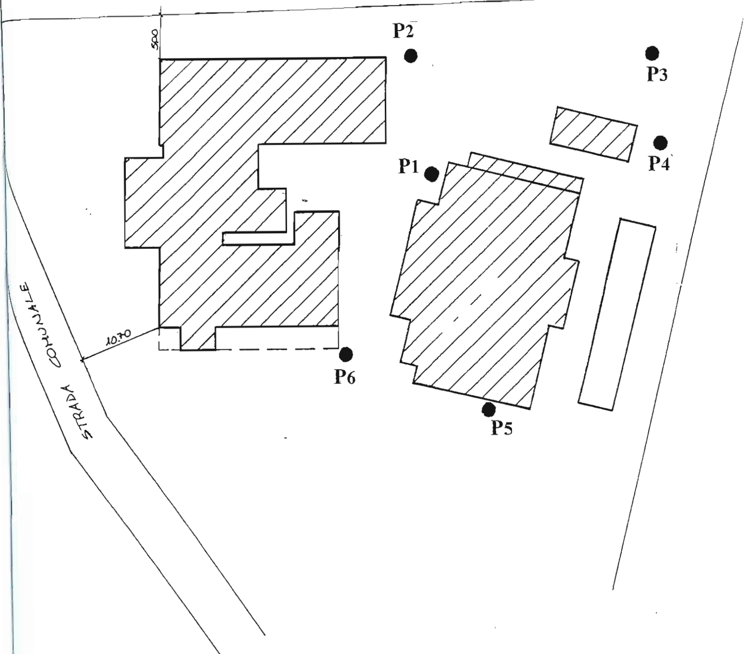
PLANIMETRIA DELLO STATO ATTUALE IN SCALA 1 : 500 CON UBICAZIONE DELLE PROVE PENETROMETRICHE
