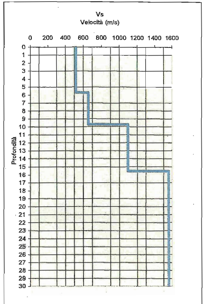
Profilo velocità/profondità
